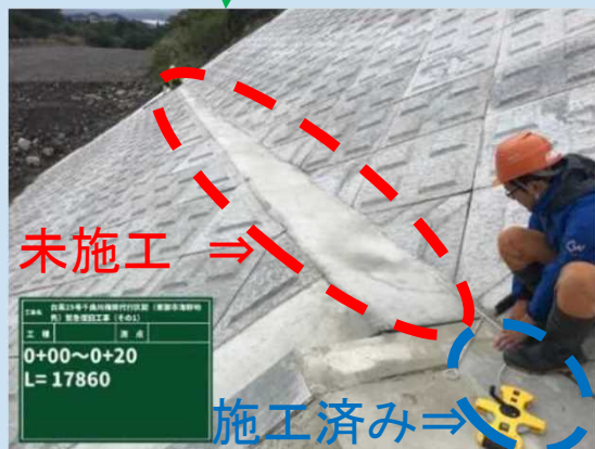
法留基礎未施工 (下流側)
