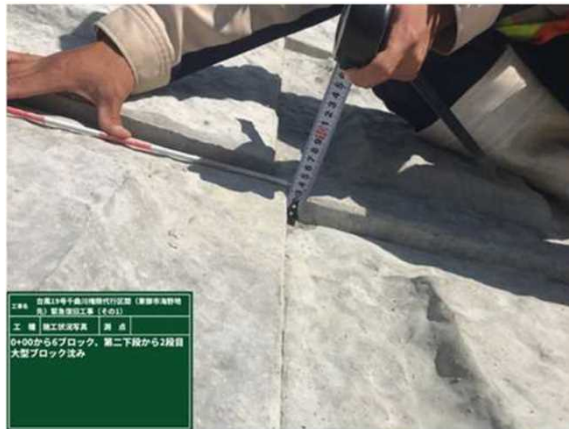
法覆大型ブロックの段差
