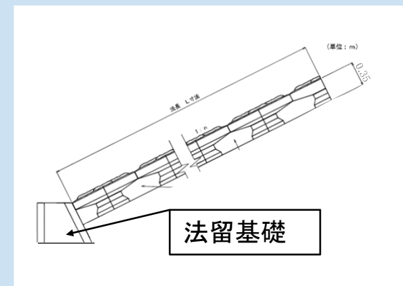
端部の処理不備 (上流側)
